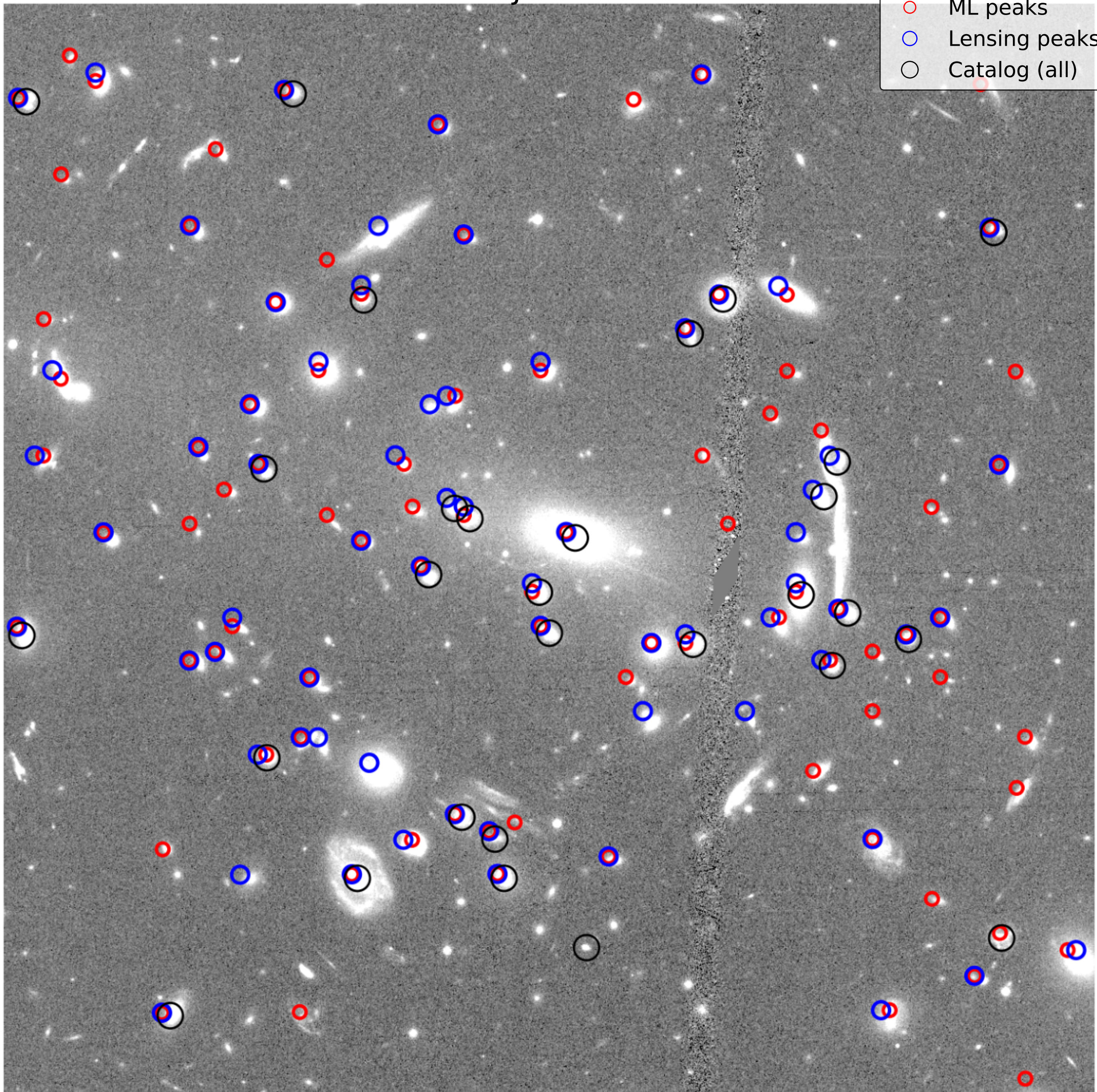
MACS J1206-0847
